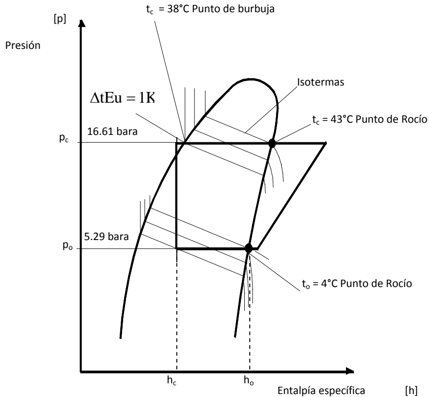
Fig. 4: Diagrama Presión - Entalpía
