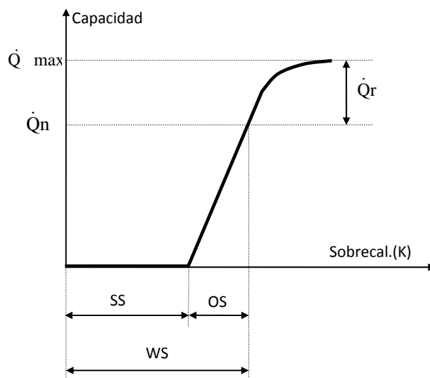
Fig.2: Diagrama de Capacidad - Sobrecalentamiento
