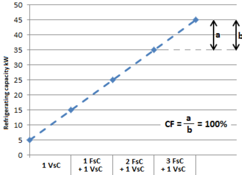
Fig. 3 : puissance frigorifique dans une centrale de compresseurs, conception optimale
