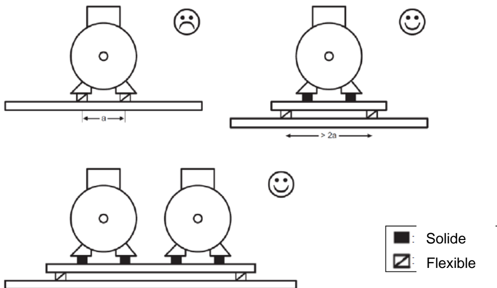
Fig. 9 : exemple de montage d'amortisseurs de vibrations
