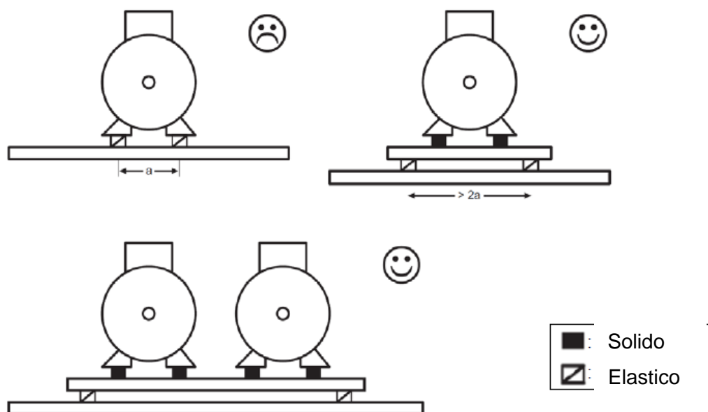
Fig. 9 - Esempio di montaggio di smorzatori antivibrazione
