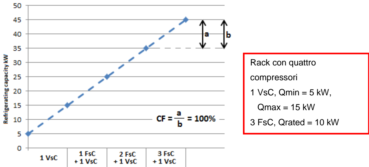
Fig. 3 – Capacità frigorifera in un rack di compressori – design ottimale
