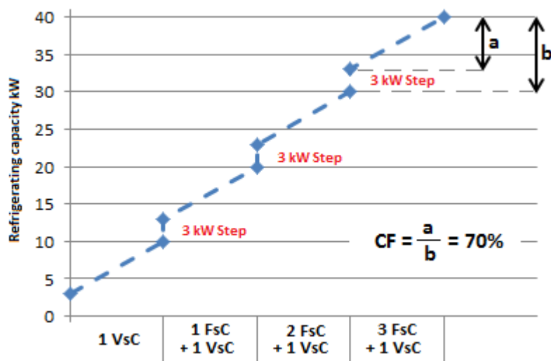
Fig. 4 – Capacità frigorifera in un rack di compressori – design non ottimale
