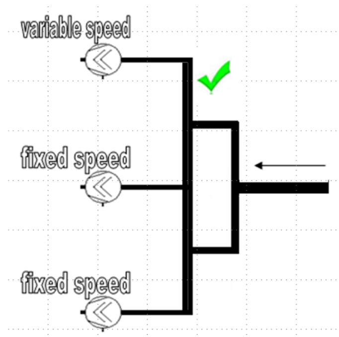
Fig 7. – Esempio alternativo di sistema correttamente progettato che può consentire di operare senza controllo del livello dell'olio
